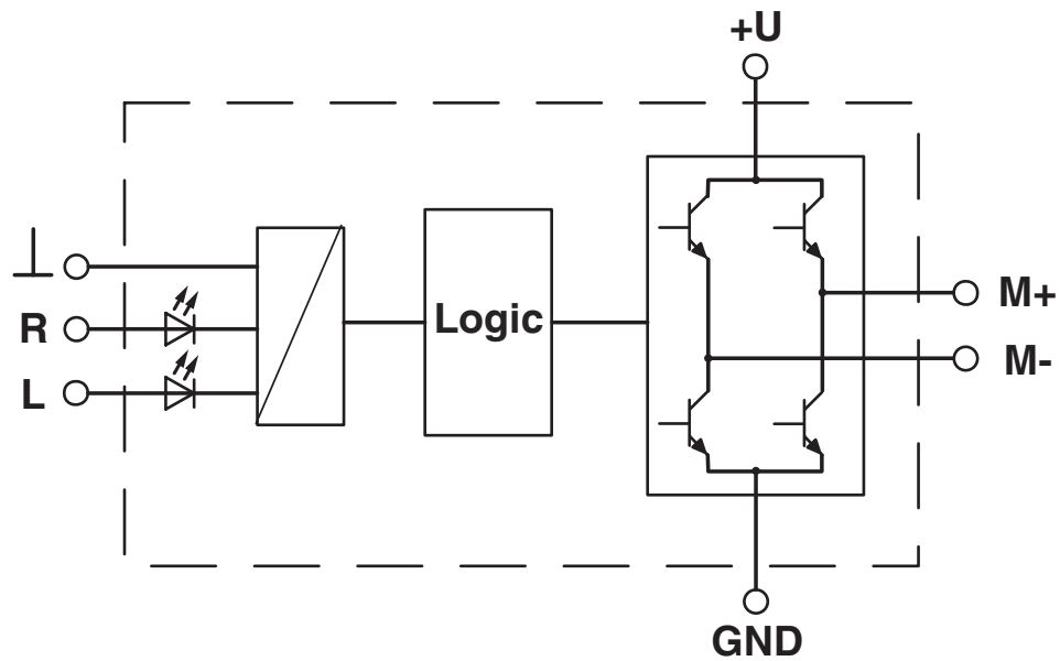
Blockschaltbild
