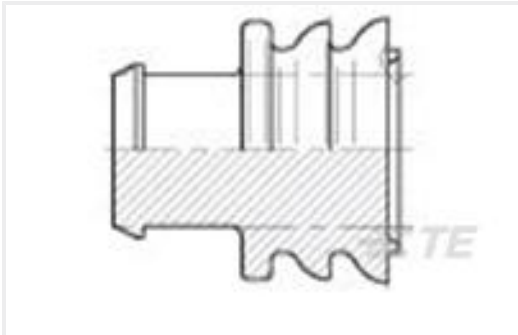
TE Part #828986-1 DICHT-STOPFEN
