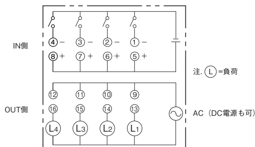
端子接続例
