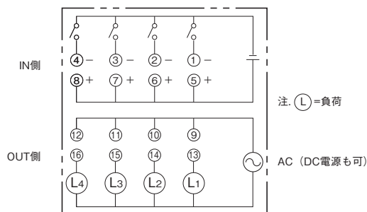
端子接続例
