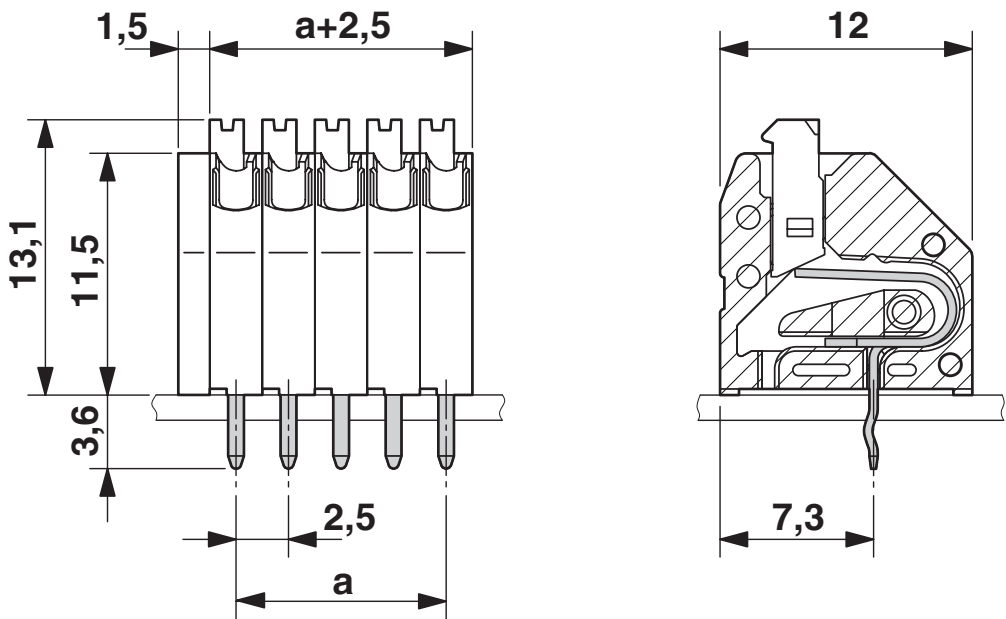
尺寸图
