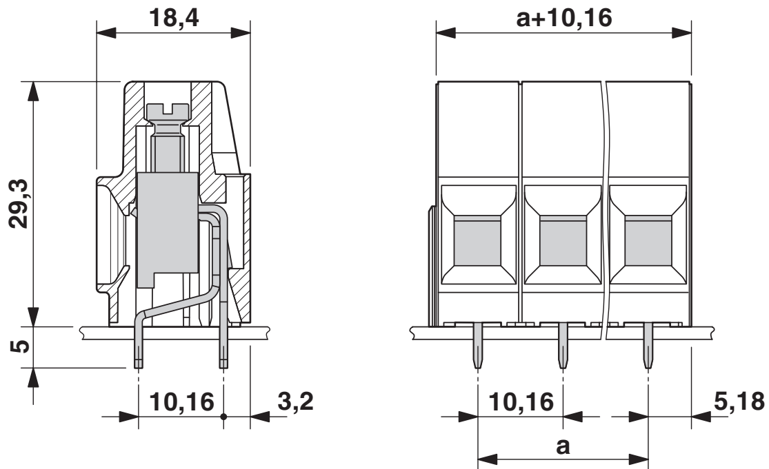
尺寸图
