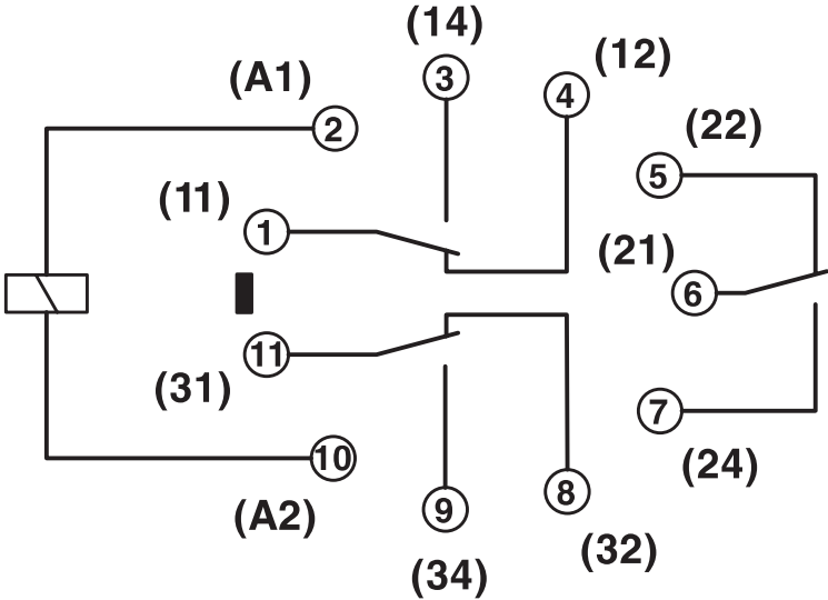
电路图
