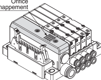
Barrette d'embase compacte mince (SS0751)
