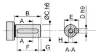
DIN 6885 A
