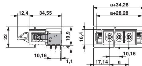
外形寸法
