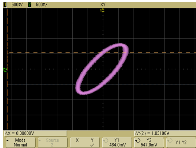
Figura 17 Cursori impostati sul centro del segnale.
