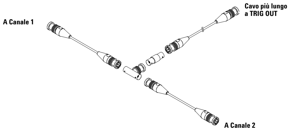
Figura 5 Cavo calibratura utente per oscilloscopio a 2 canali
