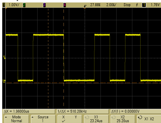
Figura 30 Spostamento dei cursori simultaneo per verificare le variazioni di larghezza degli impulsi
