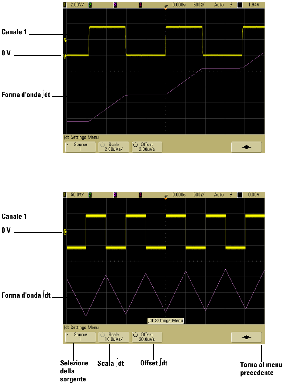
Figura 23 Integrazione e offset del segnale
