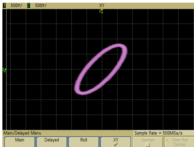
Figura 15 Segnale centrato sul display
