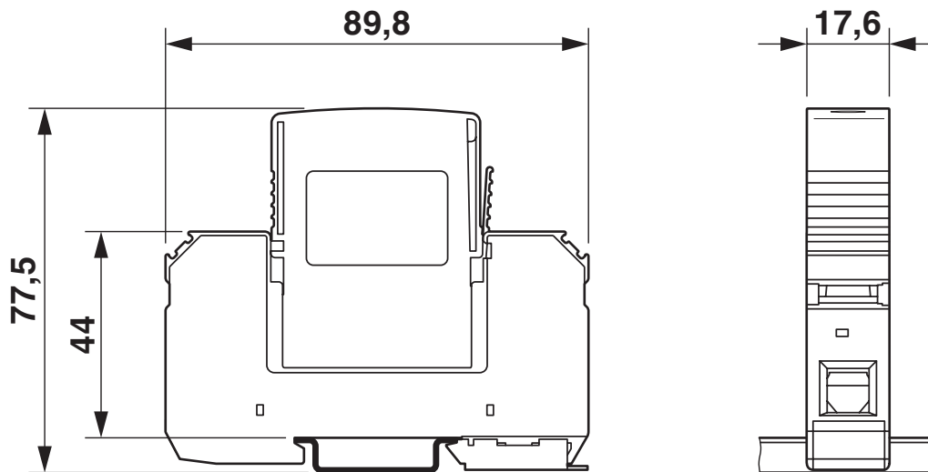
尺寸图
