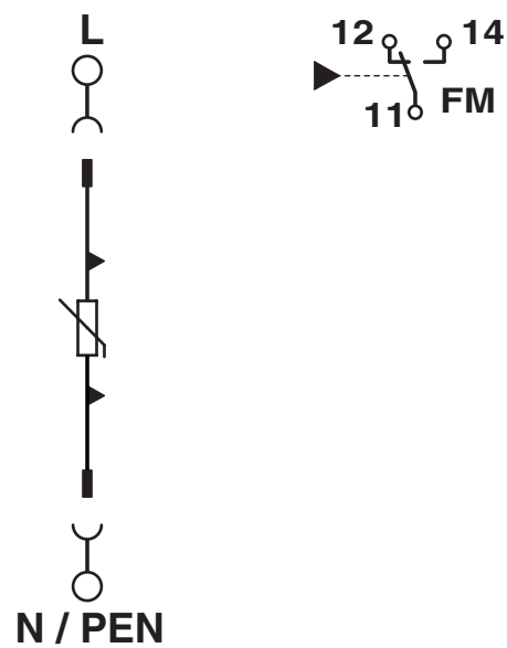
电路图
