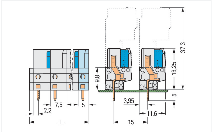
Dimensions en mm L = (\text{nombre de pôles} - 1) \times \text{pas} + 5 \text{ mm} + 1,5 \text{ mm} Connecteurs femelles à 2 pôles – seulement 1 crochet d'arrêt
