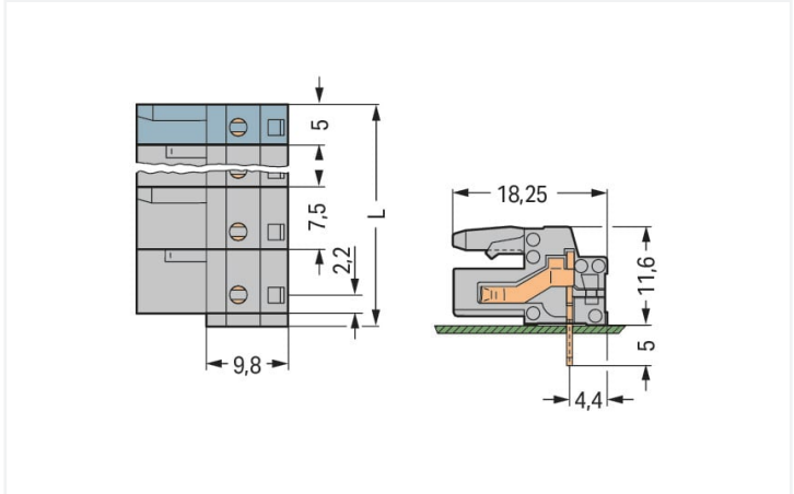
Dimensions en mm L = (\text{nombre de pôles} - 1) \times \text{pas} + 5 \text{ mm} + 1,5 \text{ mm} Distance à la première broche à souder 2,2 mm Connecteurs femelles de 2 à 3 pôles – seulement 1 crochet d'arrêt
