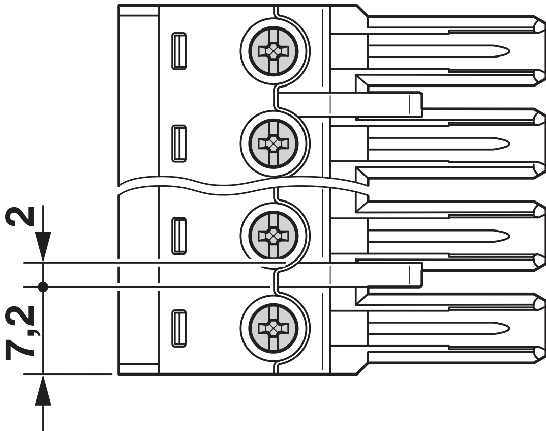
尺寸图
