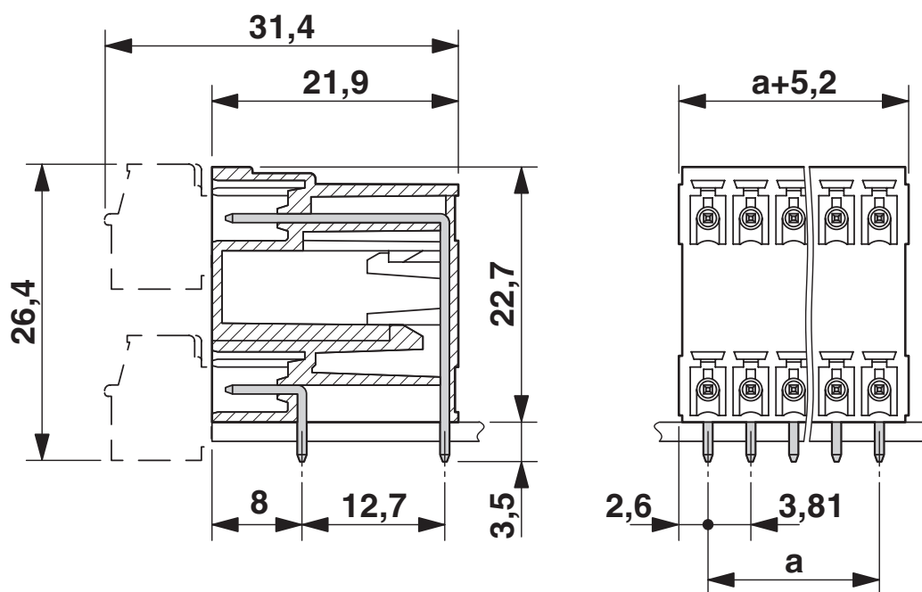
尺寸图
