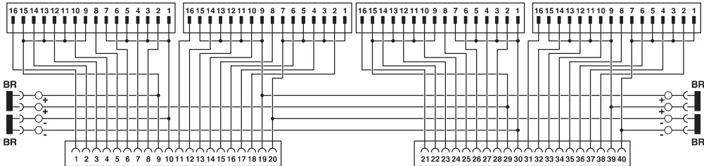
数字式西门子S7前端插入式模块6ES7 921-5AB20-0AA0或6ES7 921-5AH20-0AA0的针位分配
