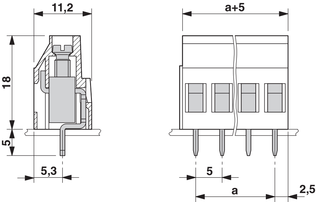
尺寸图
