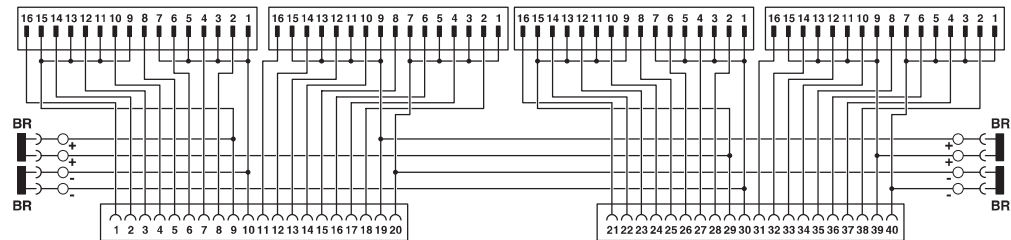
电路图
