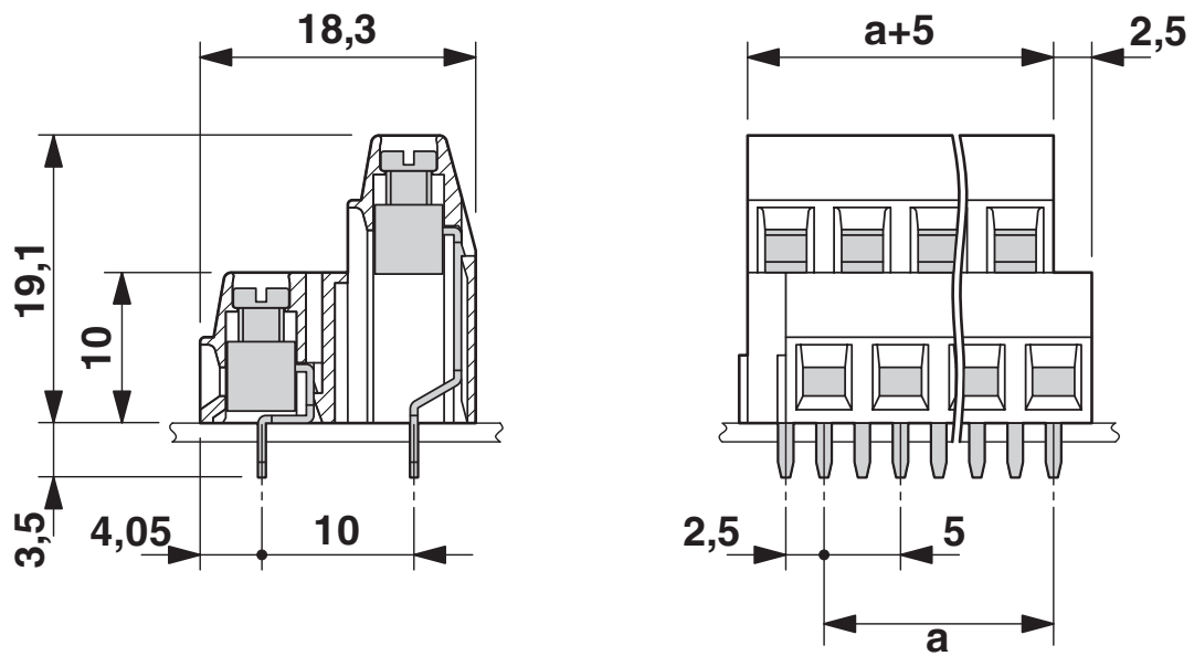
Maßzeichnung
