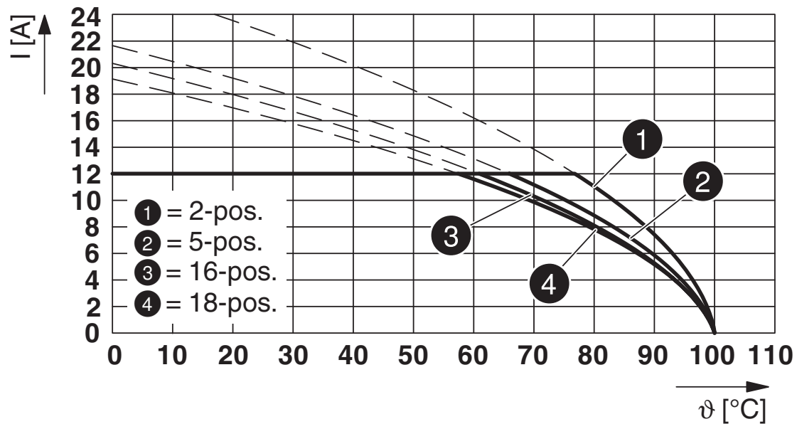
Typ: FKCT 2,5/...-ST mit FKIC 2,5/...-ST
