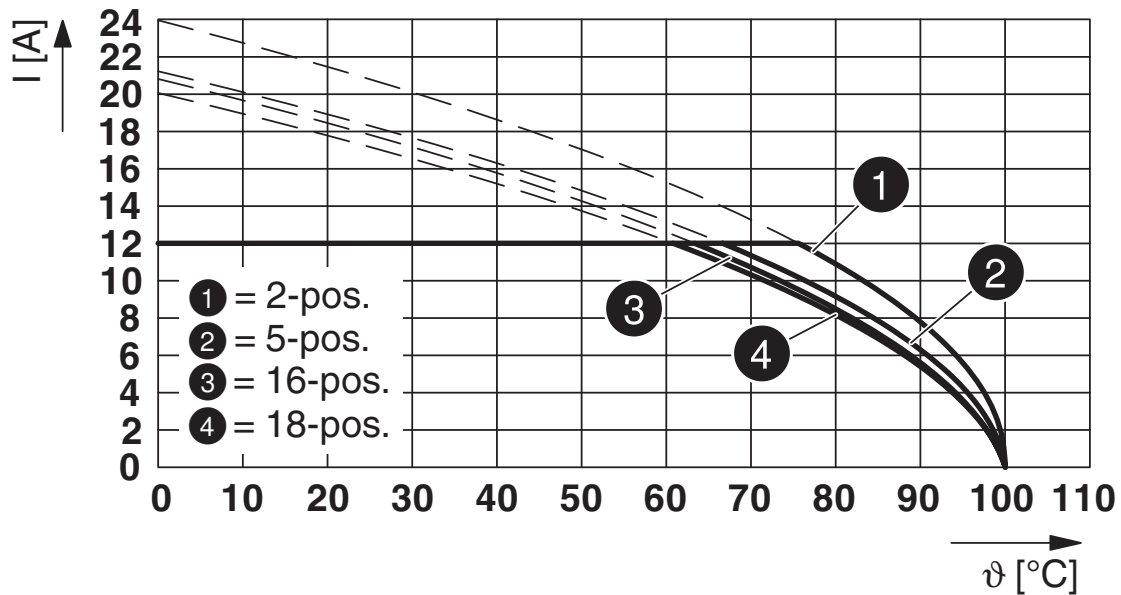
Typ: MVSTB(R/W) 2,5/...-ST mit FKIC 2,5/...-ST
