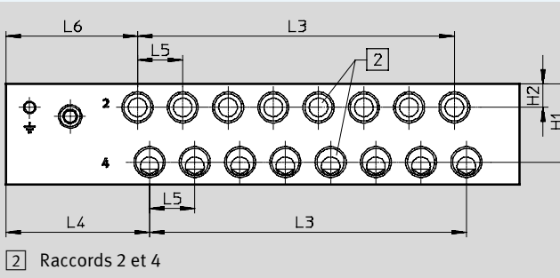
Taille 18, interface I-Port, sortie sur le dessus
