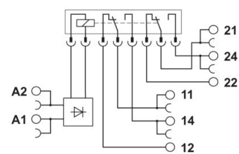
电路图
