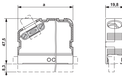
Dessin coté
