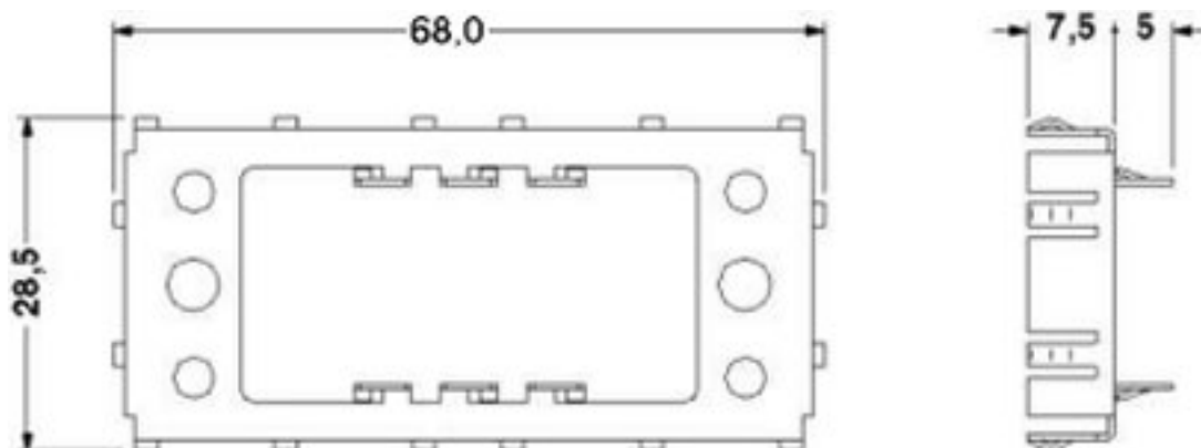
外形寸法
