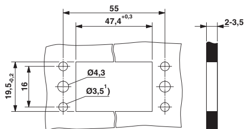
外形寸法
