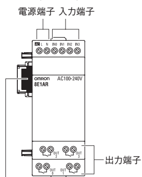
〈正面図〉
