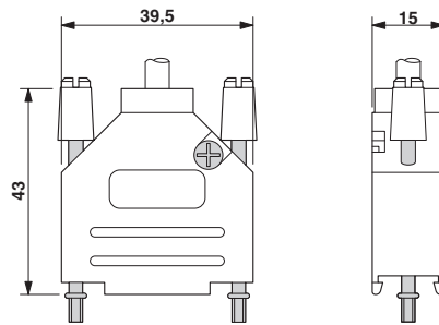
Disegno quotato
