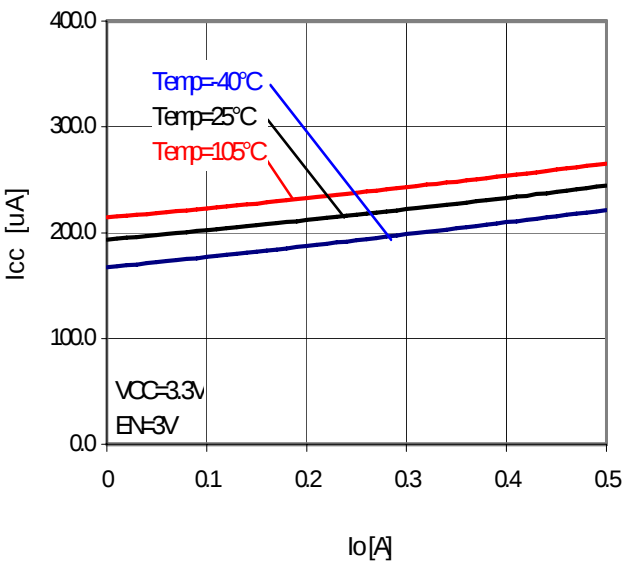
Fig.30 I_o-I_{cc}
