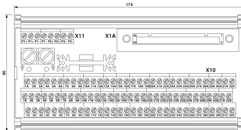
外形寸法
