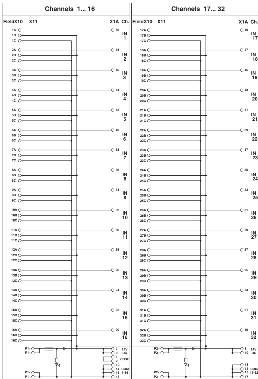
回路図
