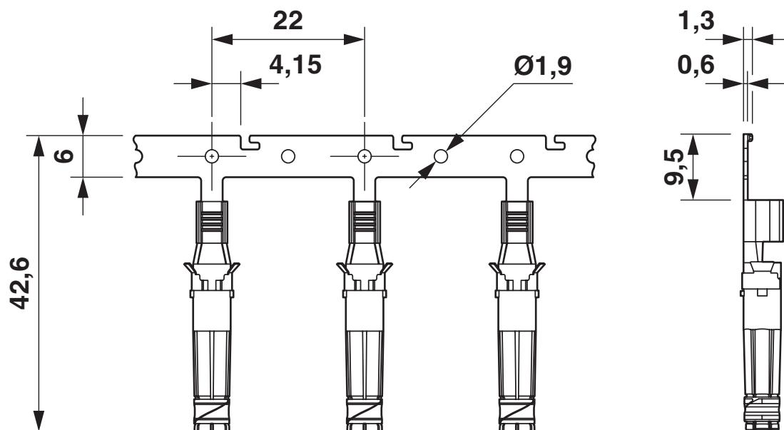
外形寸法
