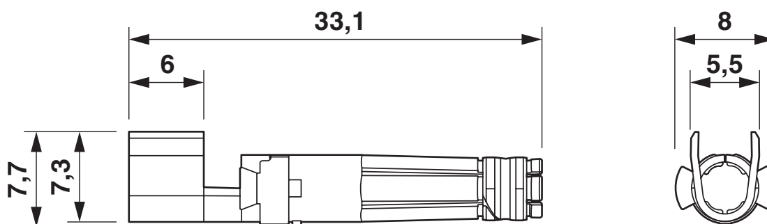
外形寸法
