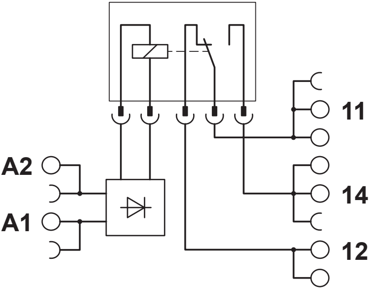
电路图
