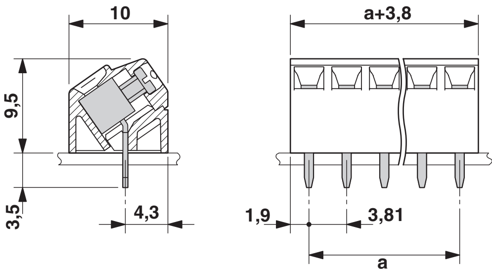
尺寸图
