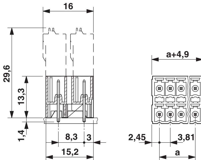
尺寸图
