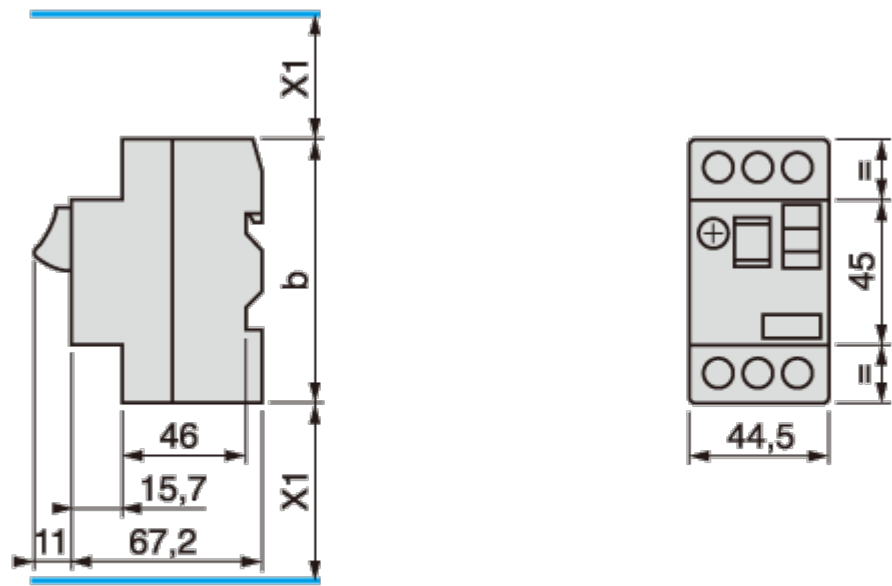
GV2ME
