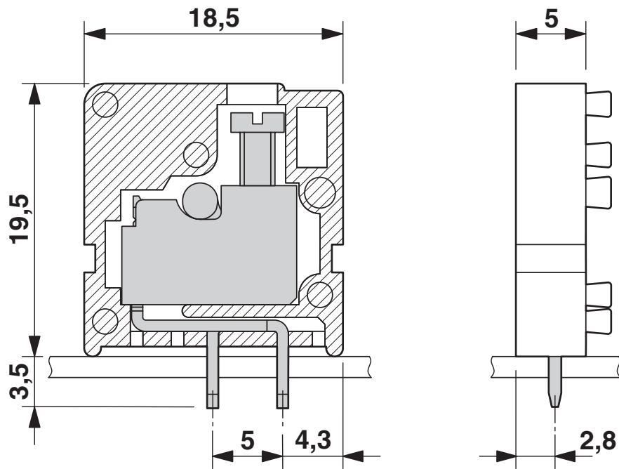
尺寸图
