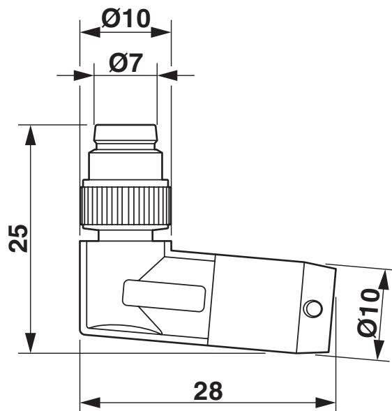
Maßzeichnung
