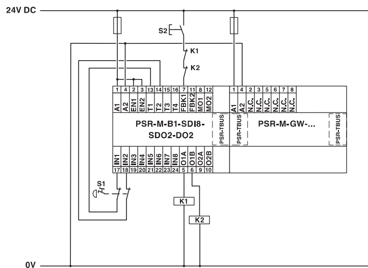
应用图
