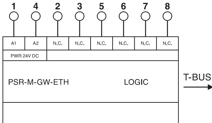
结构框图
