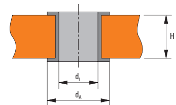
PCB parameters
