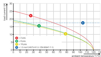
BCF 3.81../180 - SC 3.81../180
