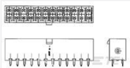
TE Part #1586037-2 2P VERT HDR VAL-U-LOK V2
