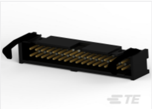
TE Part # 1-1761606-1 IDC LOW PRO HDR 34P VERT LAT BLK
