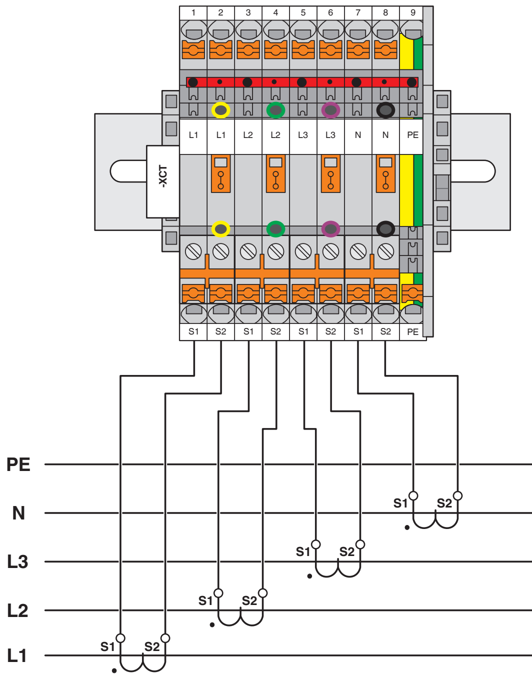
电路图
