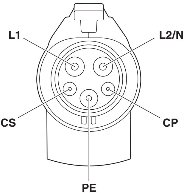
接线图
