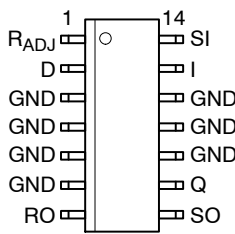
SO-14
