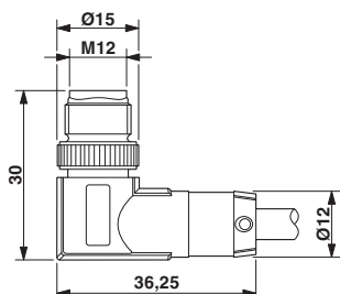
外形寸法
