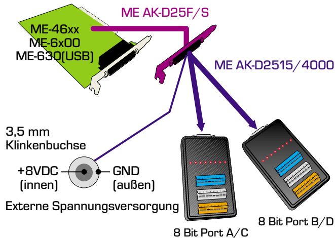
Abb. 4: Anschluß ME-Karten mit ST2
