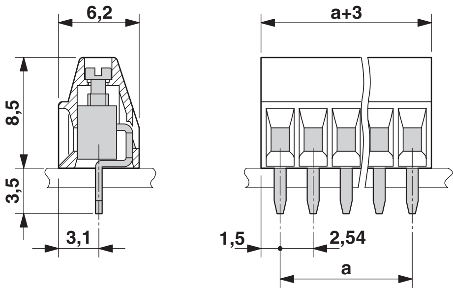
尺寸图
