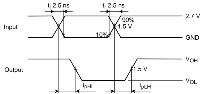
図 2 t_{pLH} , t_{pHL}
