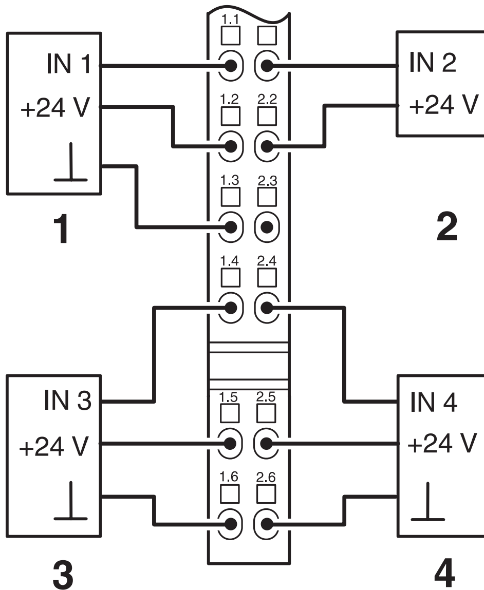
接线图
