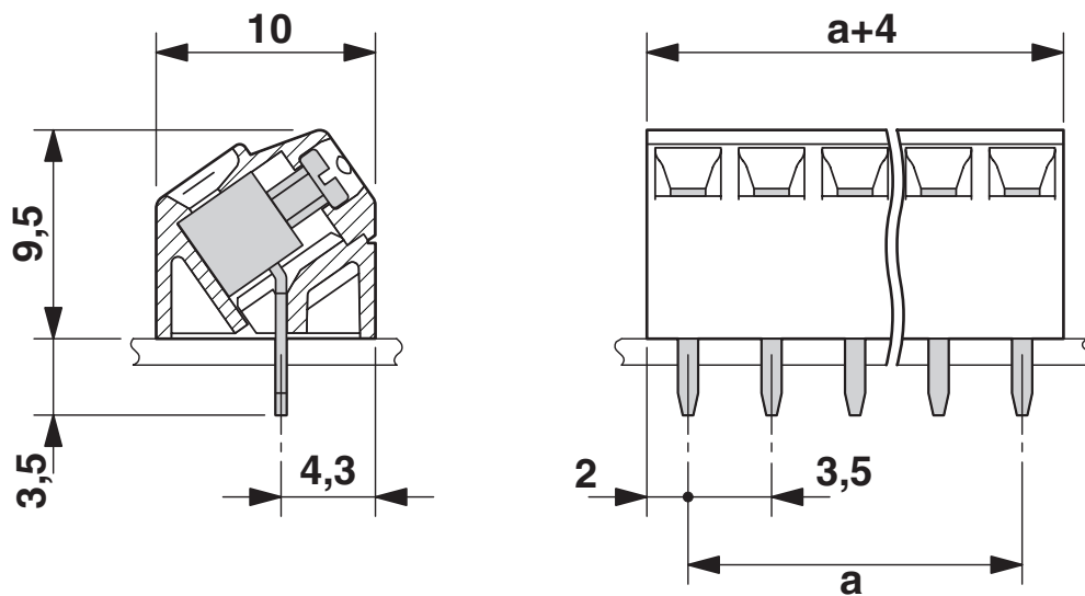
尺寸图
