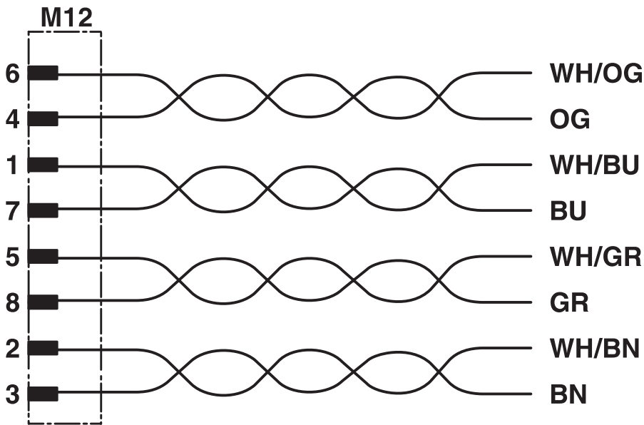
电路图
