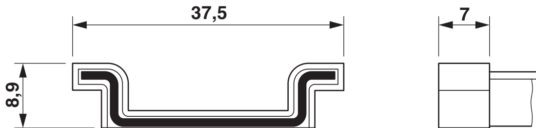
尺寸图
